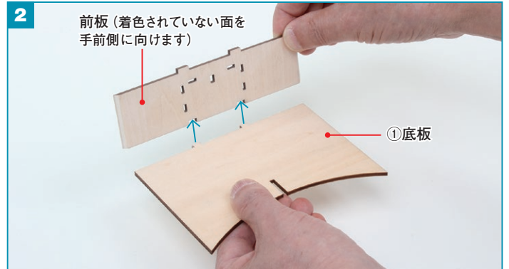
①底板の突起と前板の切り込みをかみ合わせ、ボンドで接着します。
