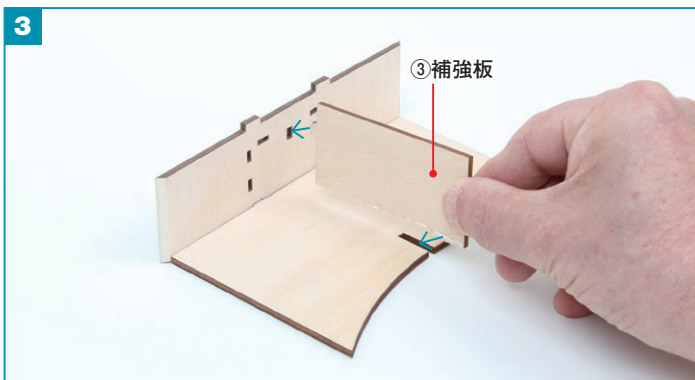
③補強板の突起を底板と前板の切り込みにはめ込み、ボンドで接着します。
