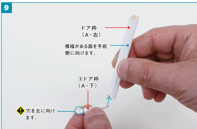
ドア枠 (A・右) に、⑨ドア枠 (A・下) をボンドで接着します。
