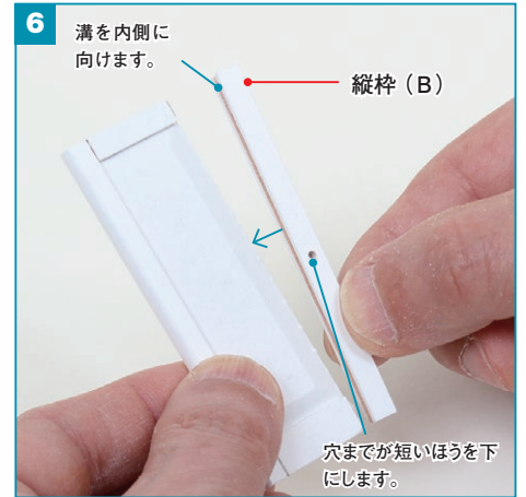
パネルの右側に、縦枠 (B) をボンドで接着します。
