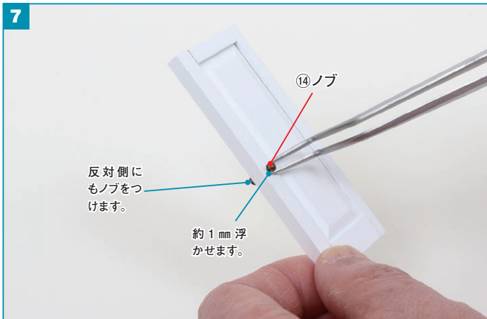
⑭ノブの端に少量の瞬間接着剤をつけ、縦枠 (B) の穴に差し込みます。
