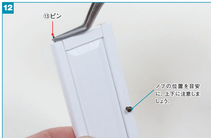
7で組み立てたドアの縦枠 (A) の上側の穴に、⑬ピンを差し込みます。
