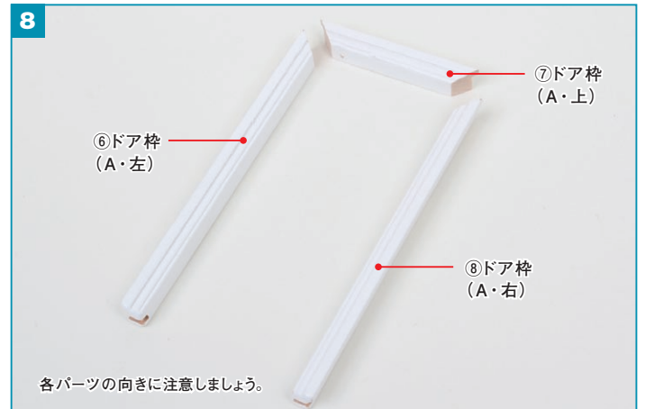
⑥ドア枠 (A・左)、⑦ドア枠 (A・上)、⑧ドア枠 (A・右) の組み合わせ方を確認します。
