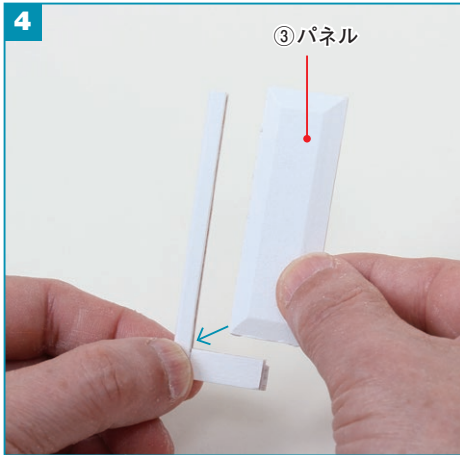
縦枠 (A) と下枠の溝に③パネルを差し込み、ボンドで接着します。
