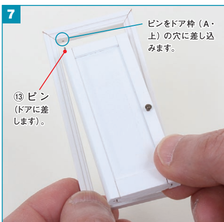
③で組み立てたドアの縦枠 (A) の上側の穴に⑬ピンを差してから、⑥で組み立てたドア枠の穴に差し込みます。
