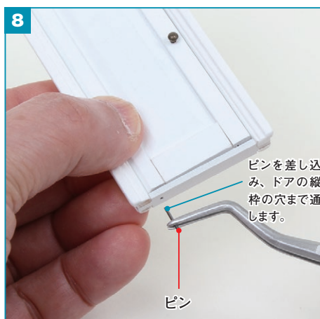
ドア枠 (A・下) の下側から残りのピンを差し込み、ドアの縦枠の穴まで通します。
