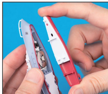
2 船体から船底を取り外します。
