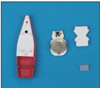
5 各パーツの取り外しが完了しました。バッテリーカバーは、船底に取り付けたままで問題ありません。
