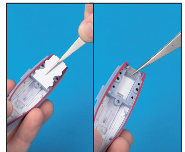
4 カーゴフロア、カーゴハッチを取り外します。ピンセットをパーツの隙間に差し込み、持ち上げるように取り外すとよいでしょう。
