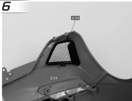
写真の2カ所に「ビス X (2.0×3mm-M)」を締め、54-4 (リアバンパーベント・右)を固定する。
