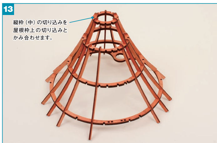
10の[13]～[16]に、縦枠(中)を1本ずつボンドで接着します。
