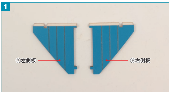
⑦左側板と⑨右側板の向きを確認します。
