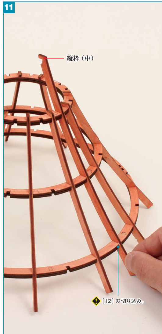
縦枠(中)の各切り込みを、10で確認した[12]の切り込みとかみ合わせ、ボンドで接着します。
