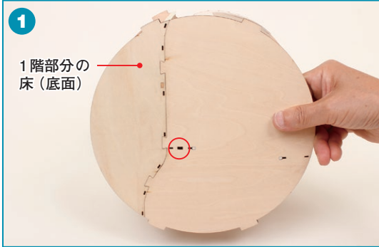
1階の床の底面、赤丸の位置の穴を確認します。
