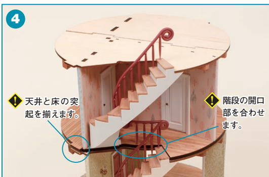
1階の天井の上に2階を乗せます。階段の開口部を合わせると同時に、天井と床の突起を揃えます。
