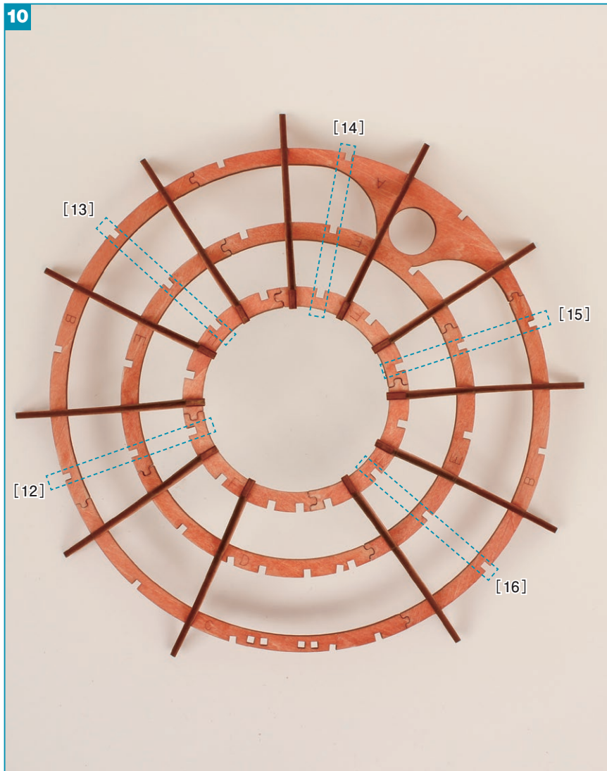
縦枠(中)を組み合わせる位置を確認します。ここでは、組み立ての目安として[12]～[16]の番号を振っています。
