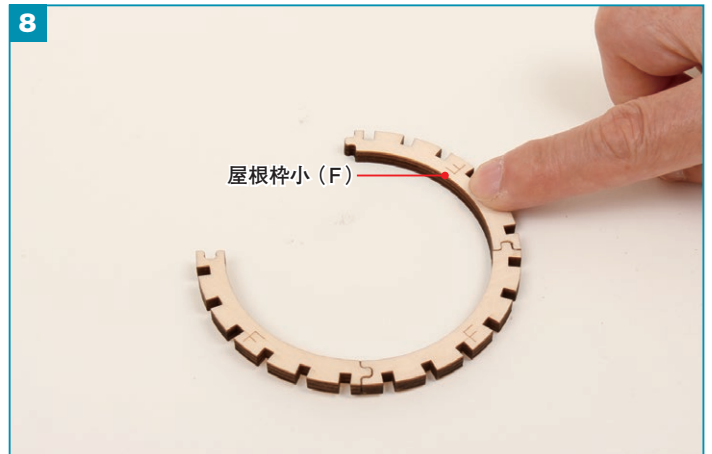
同様に、もう1本の屋根枠小 (F) の切り込みを突起とかみ合わせ、ボンドで接着します。
