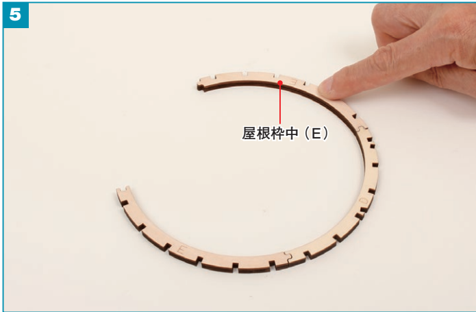
屋根枠中 (D) の反対側に、もう1本の屋根枠中 (E) をボンドで接着します。
