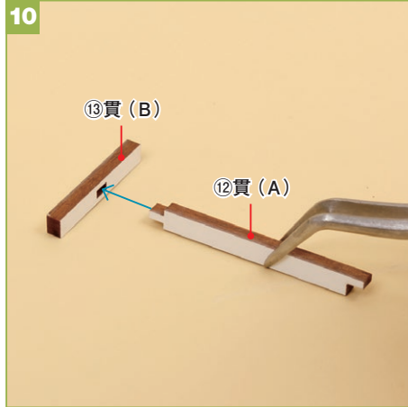
10 ⑫貫(A)の端の突起を⑬貫(B)の穴に差し込み、ボンドで接着します。
