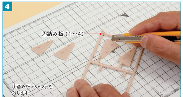
③踏み板（1～4）、④踏み板（5～8）の継ぎ目をカッターナイフで切って外し、切り口に紙ヤスリをかけて平らにします。
