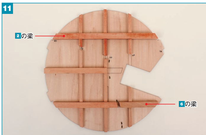
同様に2と6の梁をボンドで接着します。
