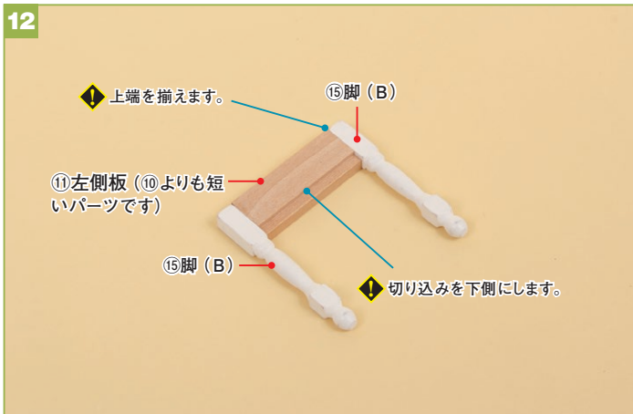
12 ⑪左側板の左右に⑮脚(B)を1本ずつ、ボンドで接着します。
