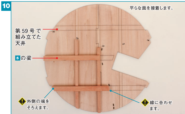
第59号で組み立てた天井を用意し、5の梁をボンドで接着します。
