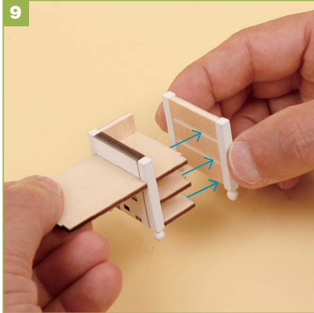
9 棚板の右側に、8で組み立てた右側面をボンドで接着します。
