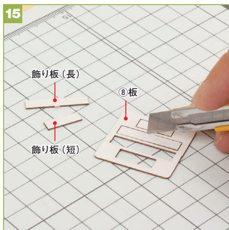
15 ⑧板の継ぎ目をカッターナイフで切って長短の飾り板を外し、切り口に紙ヤスリをかけて平らにします。
