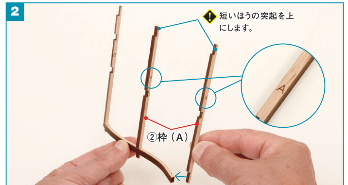
枠 (D) の残り2か所の切り込みに②枠 (A) を1本ずつ、ボンドで接着します。
