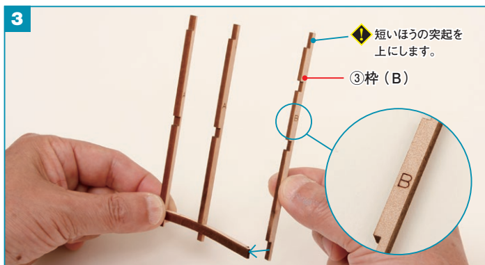
枠 (C) の右端の切り込みに、③枠 (B) をボンドで接着します。
