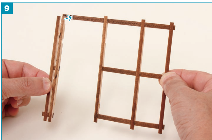
⑤で組み立てた壁枠を裏返し、左側の切り込みに⑧の壁枠をかみ合わせて、ボンドで接着します。
