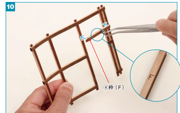
⑨の壁枠を裏返し、左右の枠の間に④枠 (F) をかみ合わせて、ボンドで接着します。
