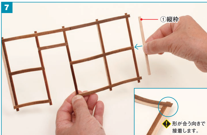
壁枠の右側に、1 縦枠をボンドで接着します。
