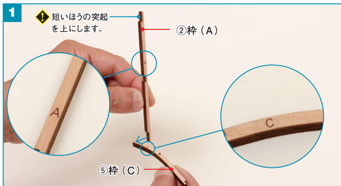
②枠 (A) と⑤枠 (C) の切り込みをかみ合わせ、ボンドで接着します。
