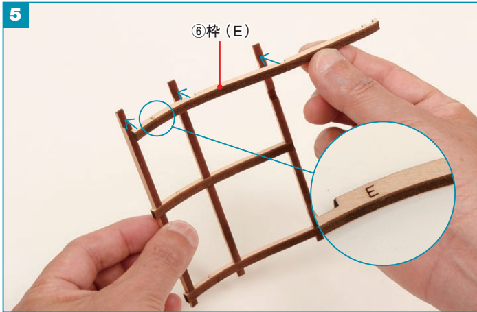
縦枠の上端の切り込みに、⑥枠 (E) をボンドで接着します。
