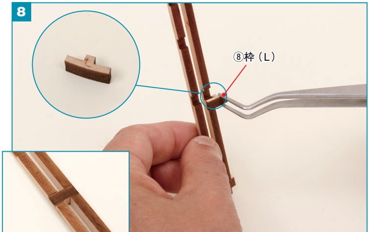
縦枠の中ほどの切り込みに、⑧枠 (L) をボンドで接着します。
