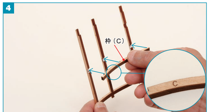
縦枠の中ほどの切り込みに、残りの枠 (C) をボンドで接着します。
