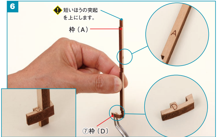
残りの枠 (A) と⑦枠 (D) の切り込みをかみ合わせて、ボンドで接着します。
