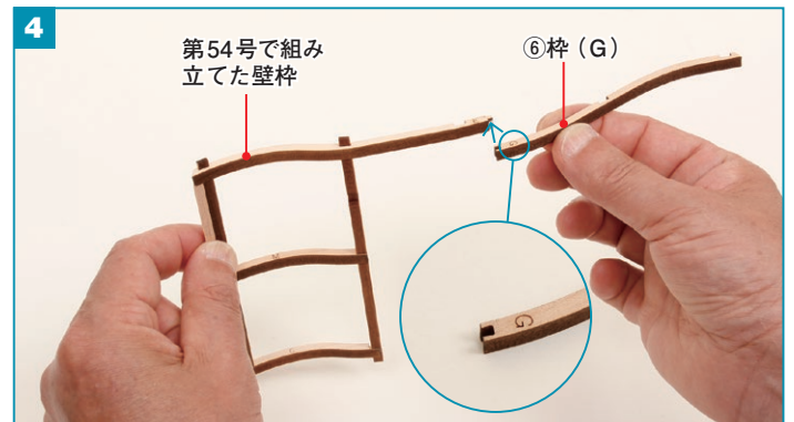
第54号で組み立てた壁枠を用意し、右側に⑥枠 (G) をボンドで接着します。
