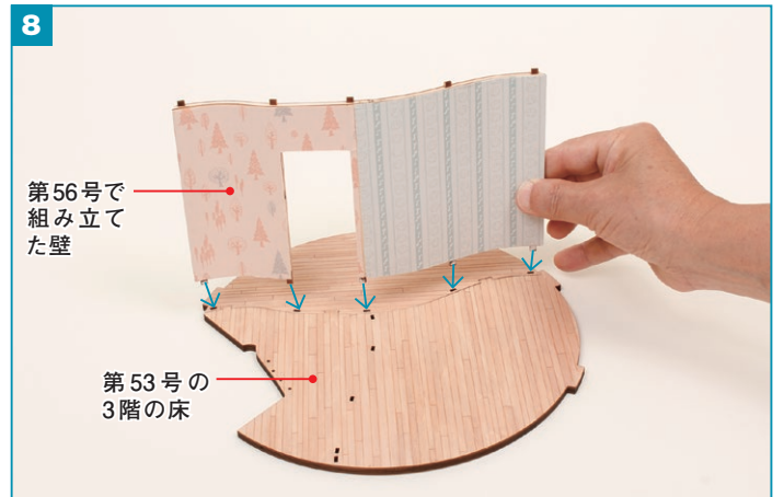
第56号で組み立てた壁の突起を第53号の3階の床の穴に差し込み、ボンドで接着します。
