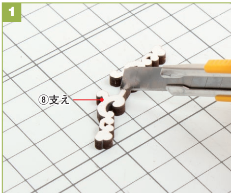
⑧支えの継ぎ目をカッターナイフで切って外します。切り口は紙ヤスリをかけて平らにします。
