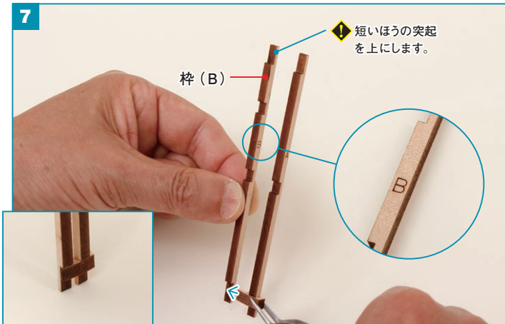
枠 (D) の左端の切り込みに、残りの枠 (B) をボンドで接着します。
