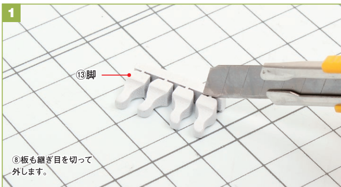
13脚(4本)と8板の継ぎ目をカッターナイフで切って外します。切り口は紙ヤスリをかけて平らにしましょう。
