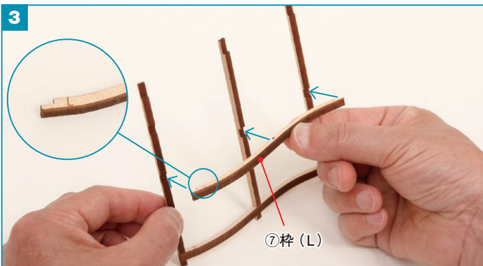
縦枠の中ほどの切り込みに、⑦枠 (L) をボンドで接着します。
