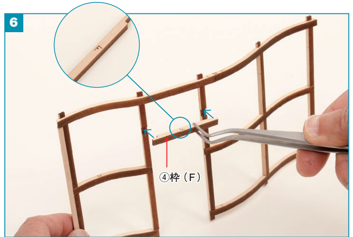
枠の中ほどに、4 枠(F)をボンドで接着します。
