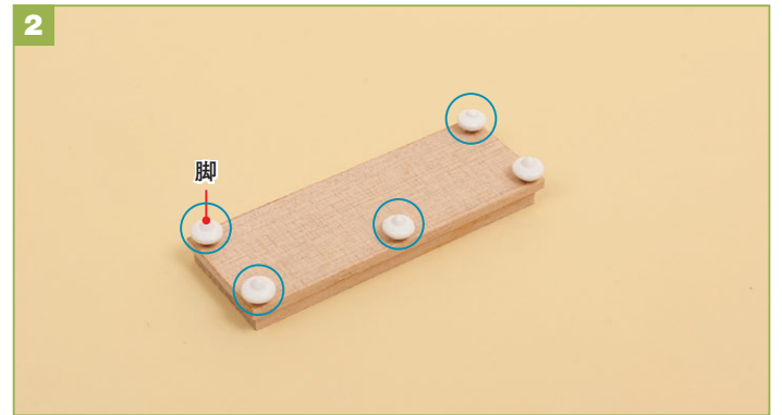
同様に、残りの穴に脚を1本ずつ、ボンドで接着します。
