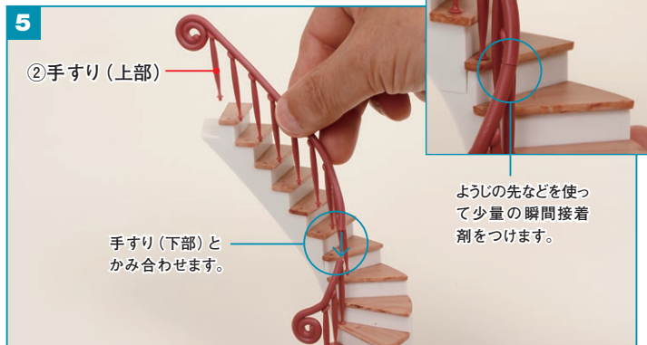
⑤ 同様に、②手すり (上部) の突起を残りの踏み板の穴に差し込み、瞬間接着剤で接着します。
