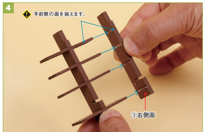
棚板の右側を③右側面の切り込みにはめ込み、ボンドで接着します。
