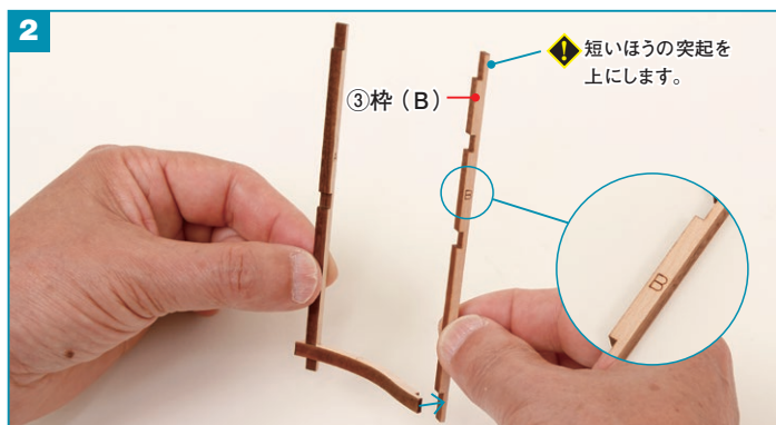
枠 (C) の反対側の切り込みに、③ 枠 (B) の切り込みをかみ合わせ、ボンドで接着します。
