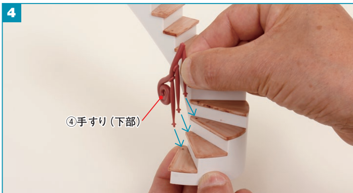
④ 手すり (下部) の突起を下から1~3段目の踏み板の穴に差し込み、瞬間接着剤で接着します。
