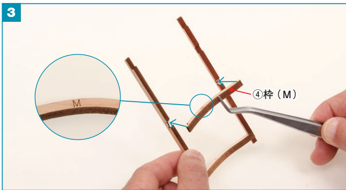
左右の枠の中ほどの切り込みに、④ 枠 (M) をボンドで接着します。
