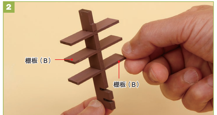
同様に、中板の上から2番目と3番目の切り込みに、棚板(B)を1枚ずつボンドで接着します。
