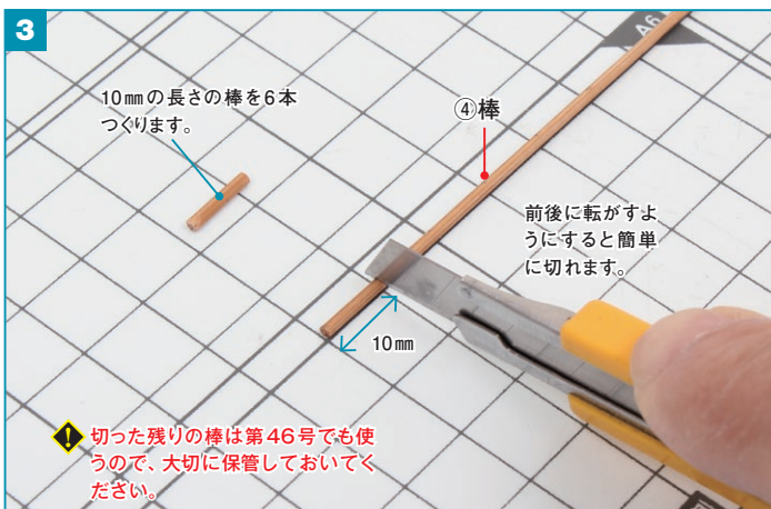
④ 棒をカッターナイフで10mmの長さに切ります。計6本用意します。
