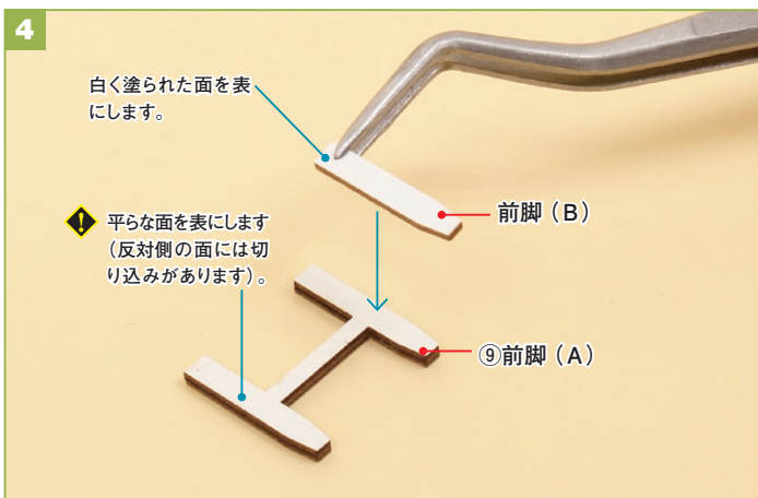
⑨前脚 (A) に前脚 (B) を1枚、形を合わせて貼ります。
