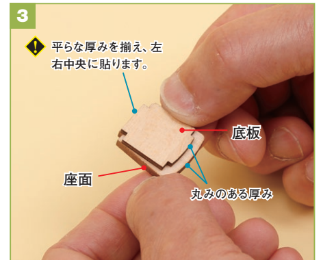
座面の底面に、底板をボンドで貼ります。
