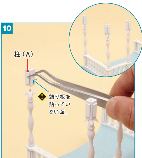
残りの円柱の上に、もう1本の柱(A)をボンドで接着します。
