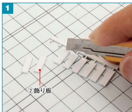
②飾り板の継ぎ目をカッターナイフで切って外し、切り口に紙ヤスリをかけて平らにします。
