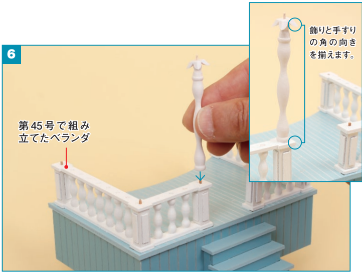
第45号で組み立てたベランダを用意し、左側の手すりの上に5の円柱をボンドで接着します。
