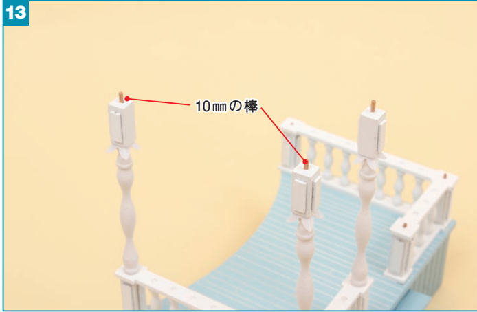
同様に、残りの柱に10mmの棒をボンドで接着します。
