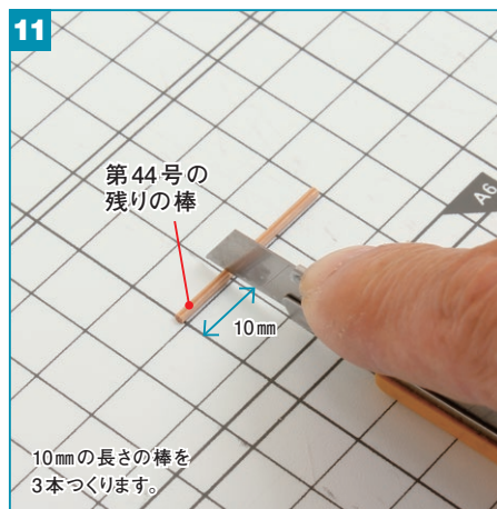
第44号の残りの棒を用意し、カッターナイフで10mmの長さに切ります。計3本用意します。
